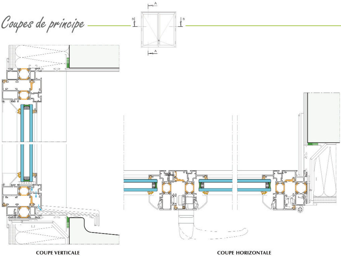
COUPE VERTICALE
